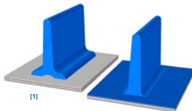
[1] Konventionel transportør [2] Hygiejnisk profilfri transportør
