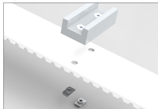
Montaggio semplice di listelli non saldati sulla cinghia a passo
