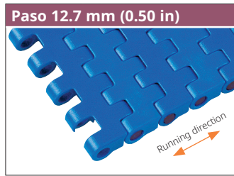
uni M-QNB Esfuerzo admisible (POM)
