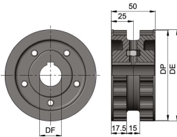
Split Sprocket
