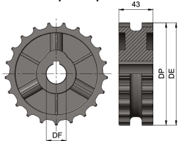
Solid Sprocket
